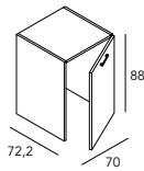
⑤ IT Modulo con anta per lavatrice / asciugatrice. EN Unit with door for washing machine/ dryer.
